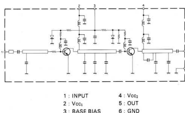
Fig. 1 Power module (V30-1131-06) Equivalent Circuit
